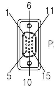
HDB15 F
